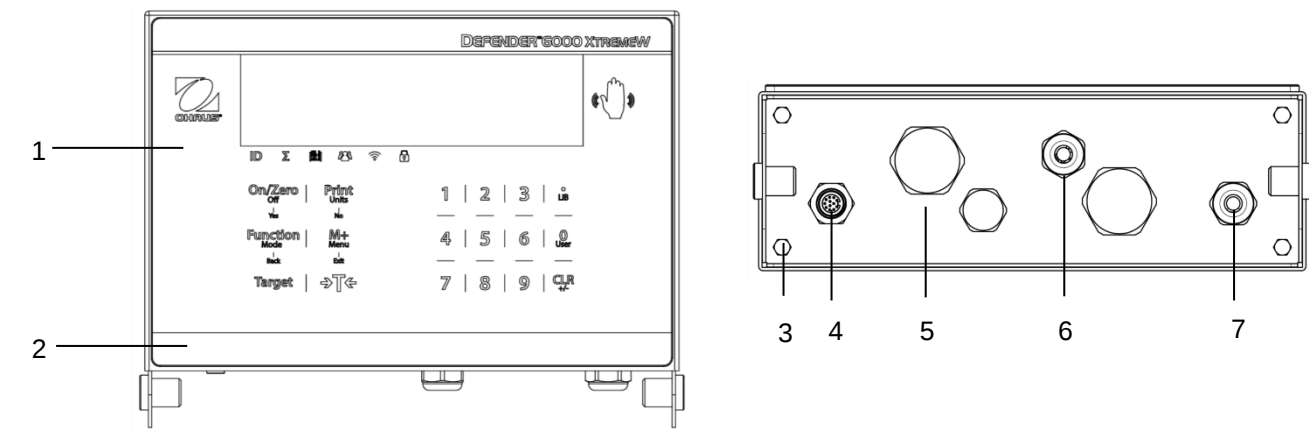
Figura 1-2 Indicador i-DT61XWE
