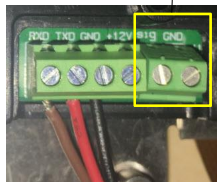
Abbildung 2-4 RS232 Stecker
