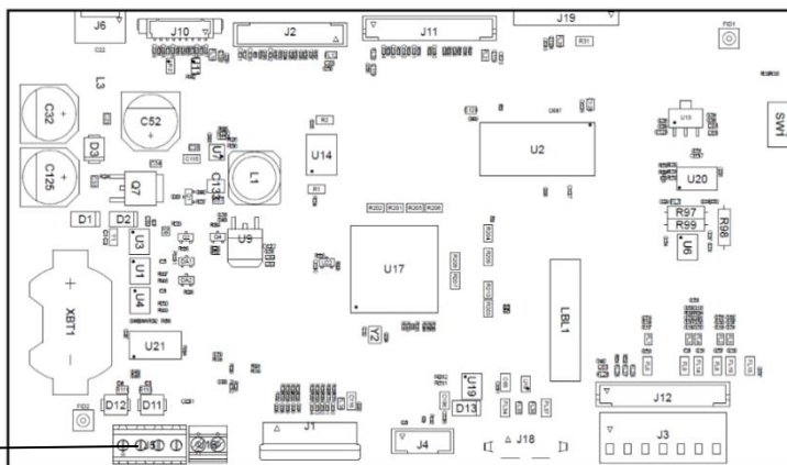
Obrázek 2-3 RS232 konektor na základní desce
