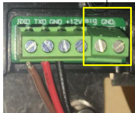
Afbeelding 2-4 RS232 stekker
