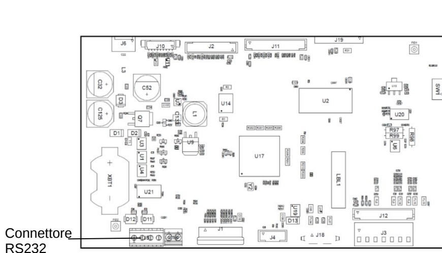
Figura 2-3 Connettore RS232 sulla scheda madre
