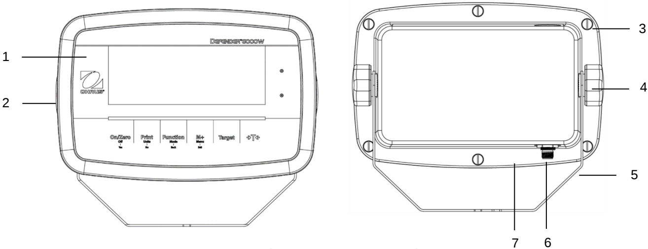
Obrázek 1-1 i-DT61PW indikátor
