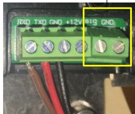
2-4 ábra RS232 csatlakozó
