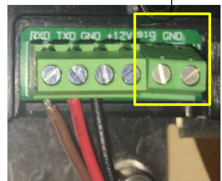
Obrázek 2-4 Konektor RS232
